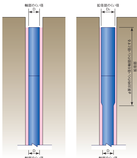
① 拡径部無しの場合
