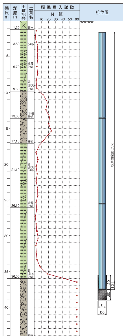
杭先端支持力
